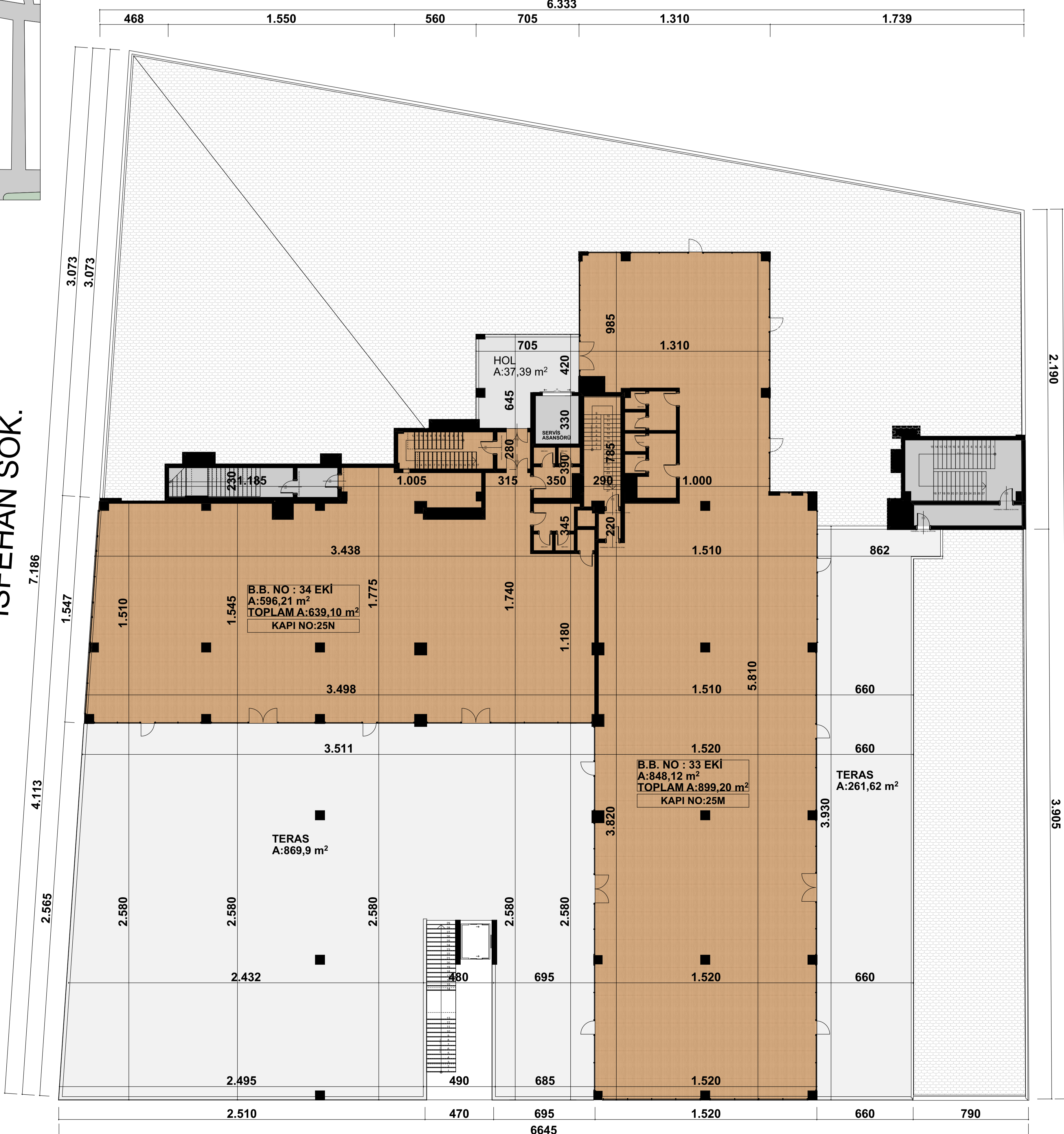
ERKAN CAD. 1. KAT PLANI
